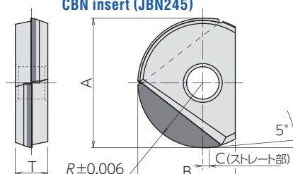
CBNチップ (材種JBN245) CBN insert (JBN245)
