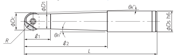
Fig.2 テーパーネック Taper neck
