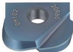
PVDコーティング(材種 JC8015 / DH102) PVD coated grade (JC8015 / DH102)
