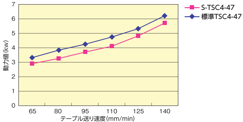
切削速度40m/min時の送り速度と動力の関係
