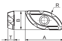
Fig.11 (外周刃)
