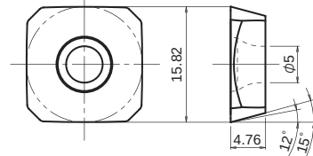
SPHW1203ZPTR
