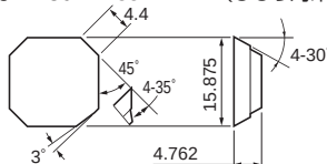
Fig.2 SGHN1504AZR-F1(びびり対策用)
