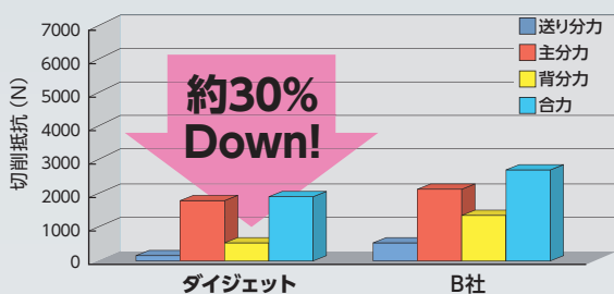
φ125, 18枚刃
