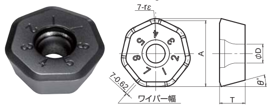
Fig. 2 プレーカなし
