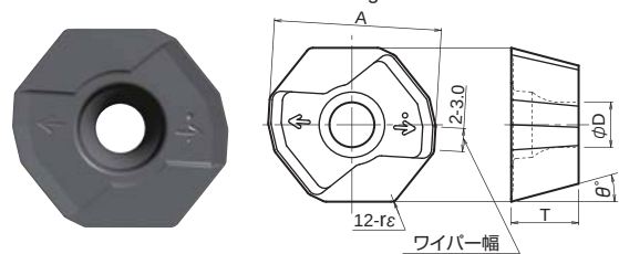
Fig. 4 さらい刃
