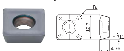
Fig.2 外周刃
