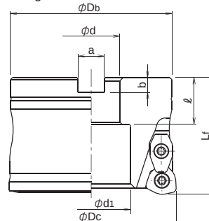
Fig.2 (クーラント穴なし)
