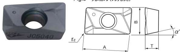
Fig.5 先端刃(刃先側)
