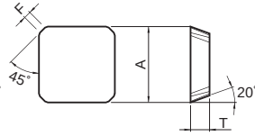
SEKN1204形 (全ての材種)
