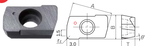
高送り用刃先強化形（EPMW100312ZTR）
