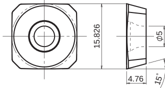
SDHW1504ADEN-F1
