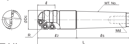
Fig.2(モールステーパシャンク)
