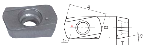
高送り用刃先強化形（EPMW100312ZTR）
