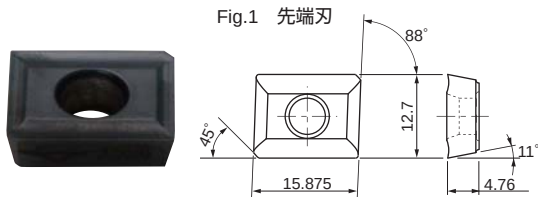
Fig.1 先端刃
