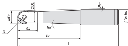
Fig.2 (テーパネック)
