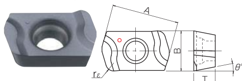
高送り用刃先強化形（EPMW100312ZER）
