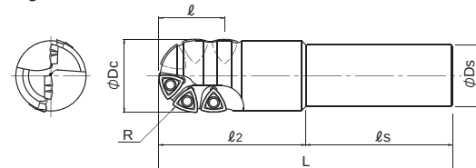
Fig.4(ストレートシャンク)
