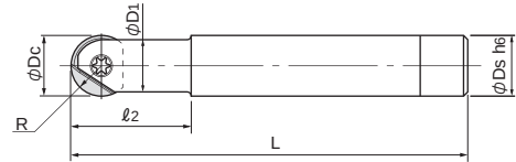
Fig.2(テーバネック)
