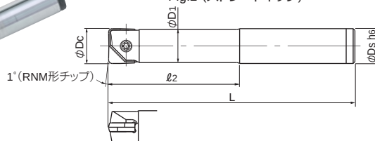
Fig.2 (ストレートネック)
