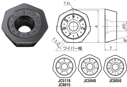
Fig. 1 プレーカなし
